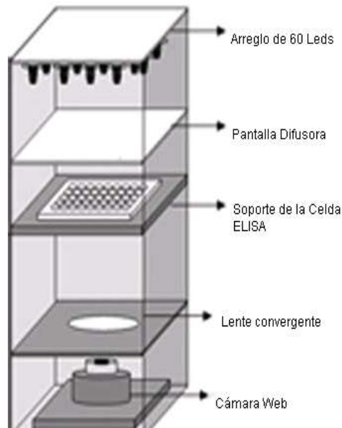
Figura 1. Esquema del diseño de un sistema colorimétrico para celdas ELISA
