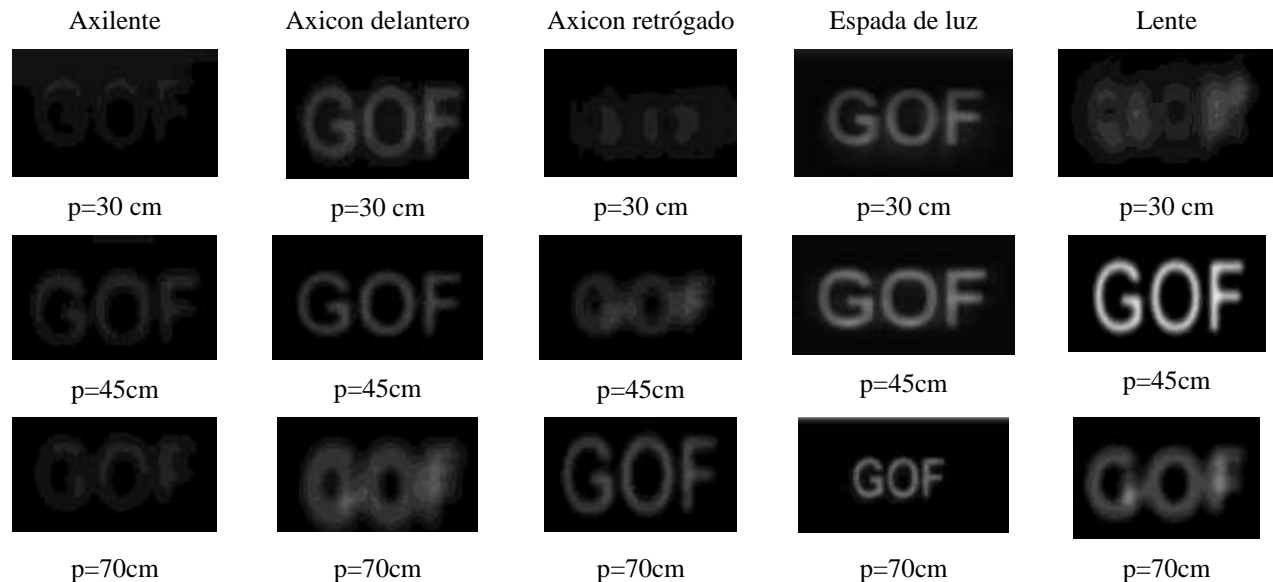
Figura 7. Imágenes producidas por los diferentes elementos ópticos difractivos de la sigla GOF colocada a la distancia mostrada debajo de cada imagen.
