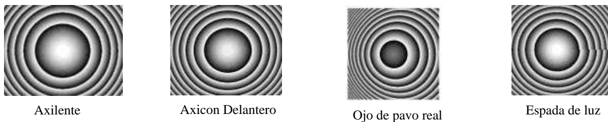
Figura 2. Representación de las transmitancias.
