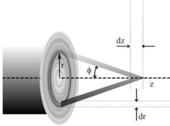
Figura 3. Diagrama que muestra el enfoque de un anillo de un axicon.
