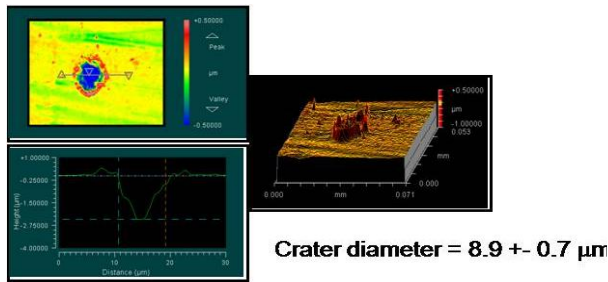
Figura 4: Micro cráteres de Ablación obtenidos a diferentes energías, empleando una longitud de onda de excitación de 1064 nm, a) 2,01 \square J y b) 47,7 \square J.
