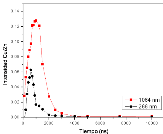
Figura 9: Intensidad de Emisión del plasma para la relación Cu I (521,82 nm) y Zn I (481,05 nm) en función del tiempo para dos distintas λ de excitación para cráteres de 7 μm generados con 200 μJ de intensidad de radiación en la condición de volumen fijo.
