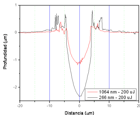
Figura 6: Perfil de Cráteres generados en la misma posición focal con la misma intensidad de radiación a dos longitudes de onda distintas.
