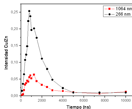
Figura 7: Intensidad de Emisión del plasma para la relación Cu I (521,82 nm) y Zn I (481,05 nm) en función del tiempo para dos distintas longitudes de onda de excitación para cráteres de 7 μm generados con 200 uJ de intensidad de radiación, en la condición de plano focal fijo.
