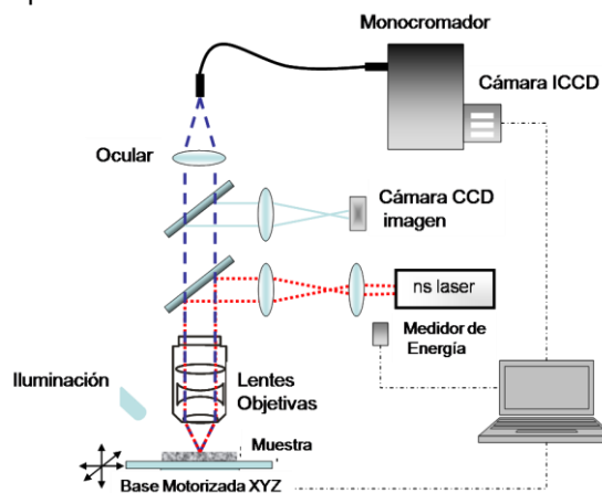
Figura 1: Diagrama del Montaje Experimental.
