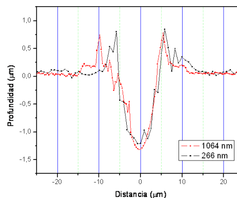
Figura 8: Perfil de los cráteres de ablación para dos longitudes de onda distintas en la condición de volumen fijo.
