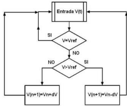
Diagrama de flujo del método voltaje constante.
