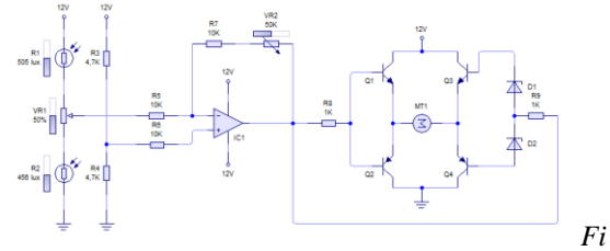
Fig. 5. Circuito de control para cada grado de libertad
