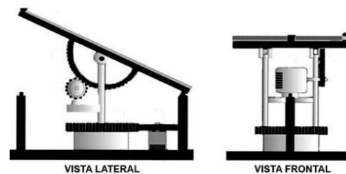
Fig. 2. Sistema seguidor solar.
