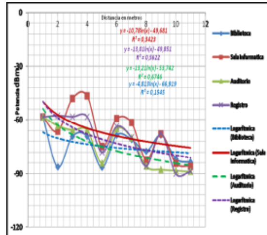
Fig. 3 (b): Curvas del modelo de regresión no lineal en Registro.
