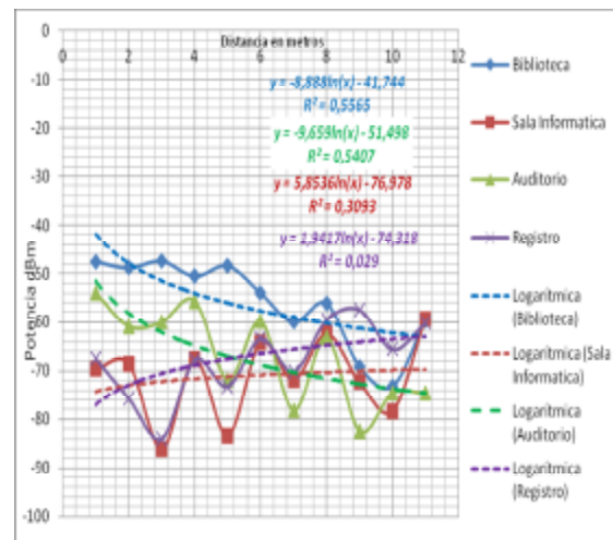
Fig.3(c) : Curvas del modelo de regresión no lineal en Biblioteca.
