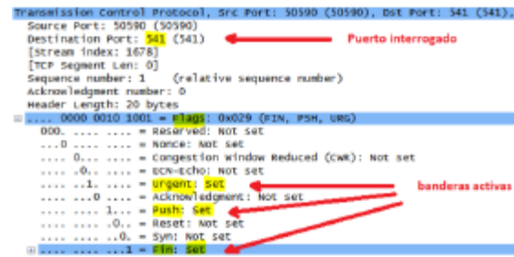
Fig. 3. TCP de un XMAS Scanning
