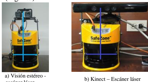
Fig. 1. Componente hardware para captación de datos.
