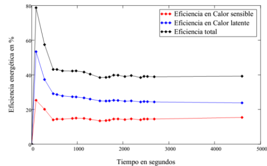
Figura 10. Eficiencia energética en % de los procesos de enfriado, secado del aire y la total en la habitación por el EAA.
