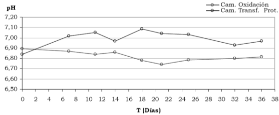
Fig. 7. Variación de pH en cámaras de oxidación y de transferencia de protones fase I. Fuente: El autor.
