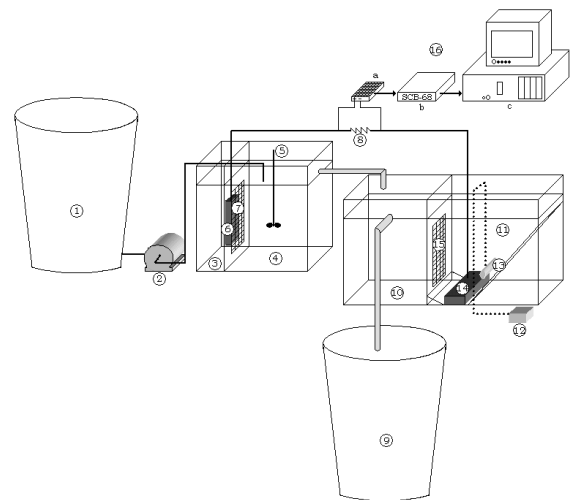
Fig. 2. Esquema y detalle del montaje inicial y del sistema de adquisición de datos implementados para la segunda fase de operación. 1.-Tanque de Agua residual, 2.-Bomba Peristáltica, 3.- Electrolito, 4.-Cámara de Oxidación, 5.- Mezclador, 6.-Anodo, 7.-Membrana Aniónica, 8.- Circuito eléctrico, 9.-Tanque para almacenar el efluente, 10.-Cámara de Transferencia de Protones, 11.-Cámara de Reducción, 12.-Aireador, 13.-Piedra Difusora, 14.-Cátodo, 15.-Membrana Catiónica y 16.-Sistema de Adquisición de datos: a) Caja de resistencias, b) Bloque Conector y c) Computador. Fuente: El autor.
