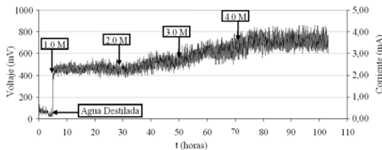
Fig. 9. Voltaje y corriente generada para diferentes concentraciones del electrolito (NaCl). Fuente: El autor.
