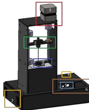
Fig. 3. Diseño del equipo de extracción de volátiles.
