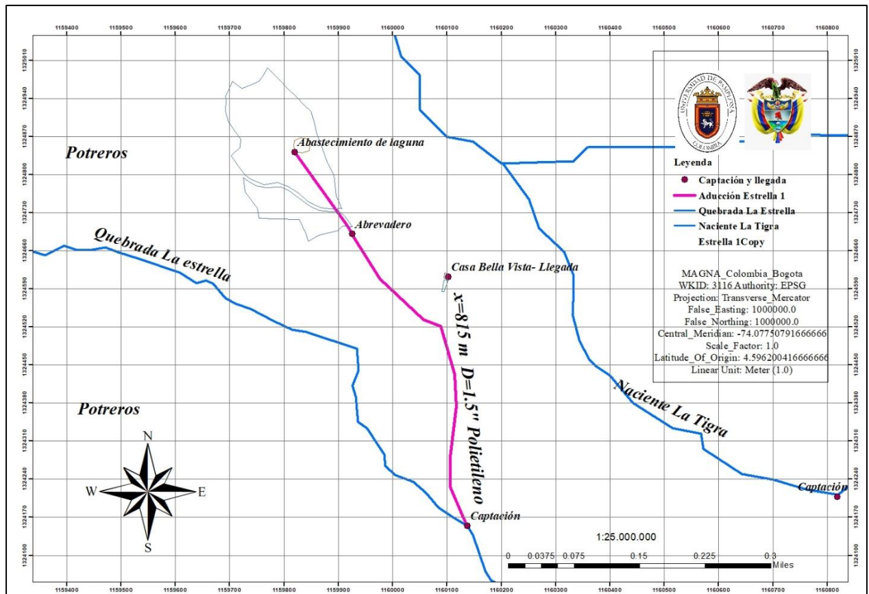
Ilustración 15. Infraestructura hidráulica.
