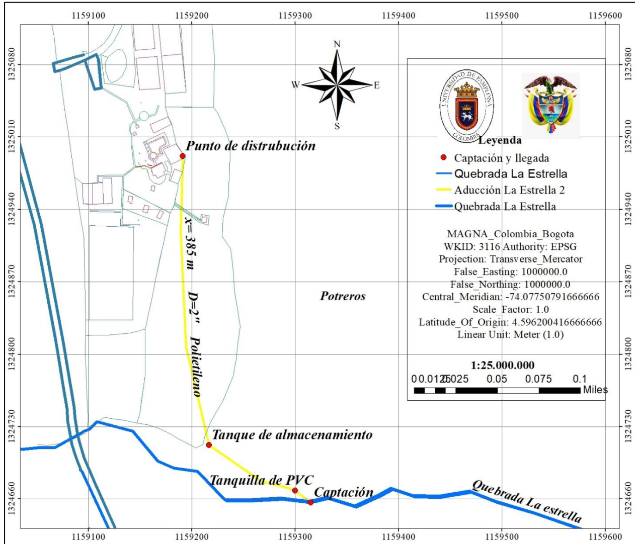
Ilustración 11. Infraestructura hidráulica.
